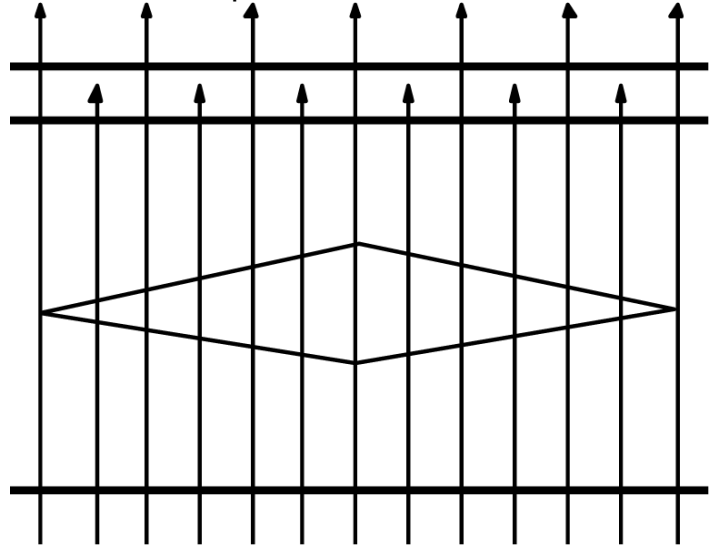
Заборная секция 2
