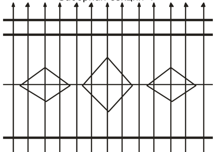
Заборная секция 4
